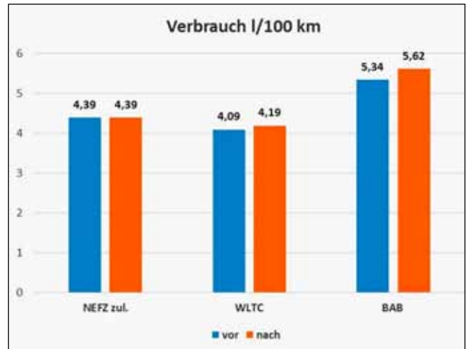
Bild 12: Entwicklung des Kraftstoffverbrauch vor und nach der Umrüstung
