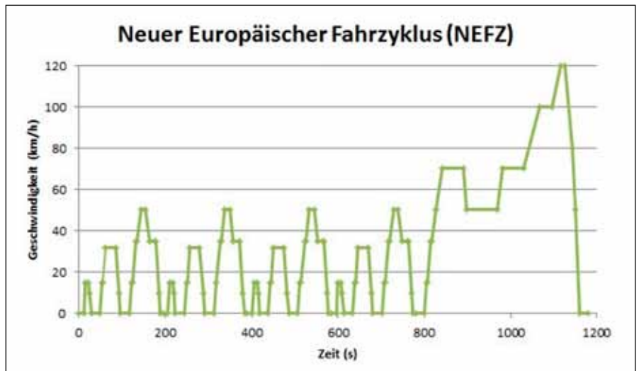
Bild 2: NEFZ Fahrzyklus
