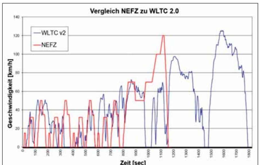
Bild 3: Vergleich neuer WLTC zu NEFZ Zyklus
