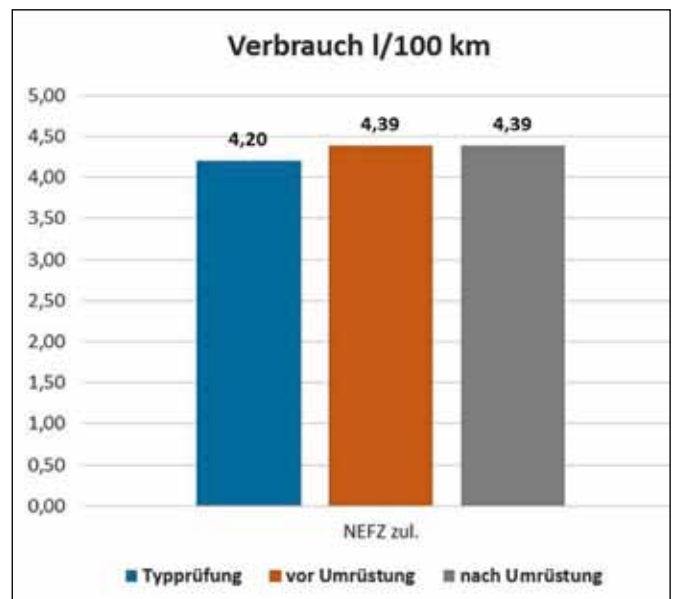
Bild 14: Vergleich Kraftstoffverbrauch Typprüfung und vor und nach der Umrüstung
