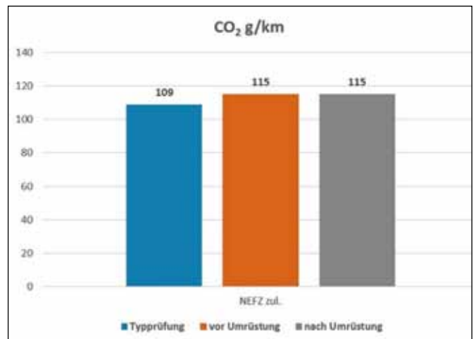
Bild 13: Vergleich des CO 2 -Wertes –Typprüfung vor und nach der Umrüstung
