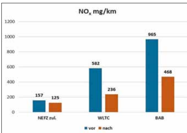
Bild 11: Entwicklung der Nox-Werte vor und nach der Umrüstung
