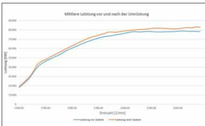
Bild 10: Mittlere Leistung vor und nach der Umrüstung
